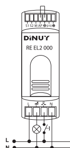
Ejemplo N° 1: con Pulsador
