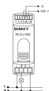
Ejemplo N° 3: con Señal 0/10Vcc
